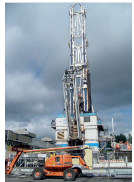
Abb. 6: Die Anger's Söhne Bohr- und Brunnenbaugesellschaft bringt mit der elektrohydraulischen Bohranlage „Innovarig“ modernste Technologie zum Einsatz
