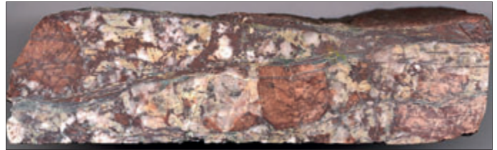
Abb. 7: Geklüftete granitische Gesteine, eine vorteilhafte Geologie für die Nutzung der Wärme aus dem Untergrund (Foto: Geothermie Soultz)
